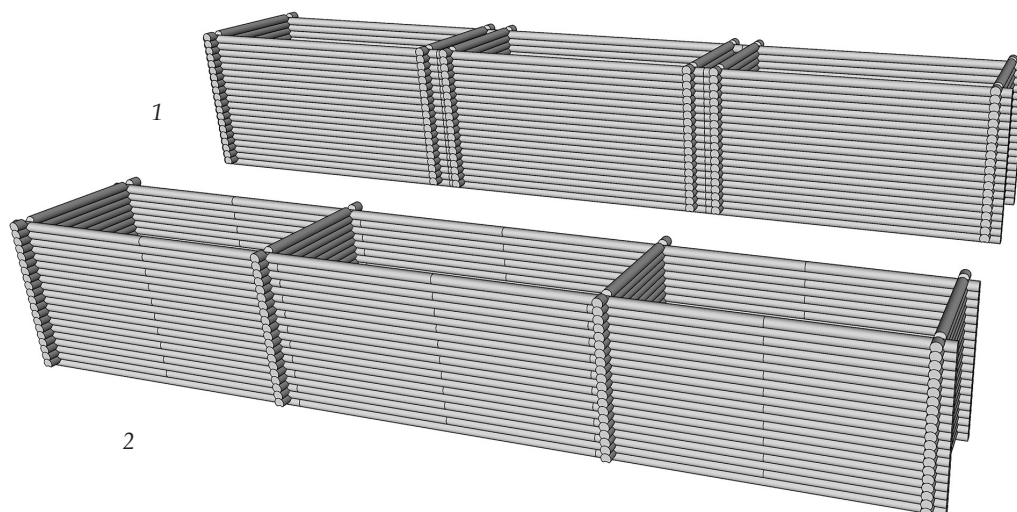
Рис. 1. Основные разновидности рубленых стен, согласно современным представлениям (показаны без мостов и обломов): 1 — городни из отдельных срубов, поставленных вплотную друг к другу; 2 — тарасы («рубленный город», городни в виде двух параллельных венчатых стен с перерубами, «в две стены» по С. В. Горохову)
