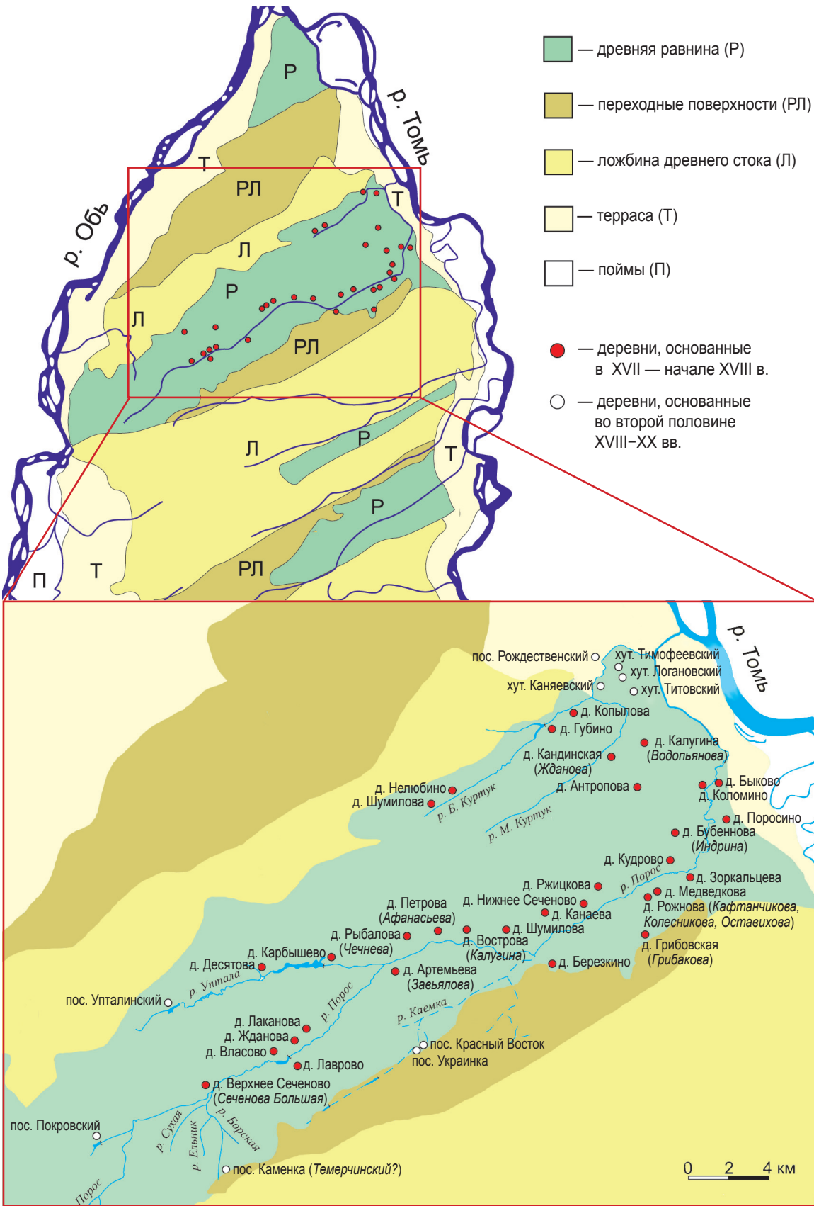
Основные типы поверхностей Обь-Томского междуречья (по: Дюкарев А. Г., Пологова Н. Н. Указ. соч. Рис. 1.) и карта-схема сельских населенных пунктов долины р. Порос
